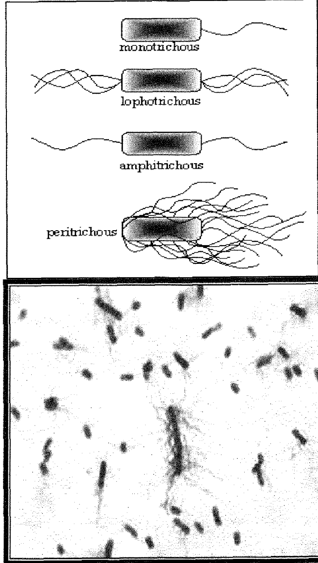
شكل (17) انواع الاسواط البكتيرية تظهر تحت المجهر .
