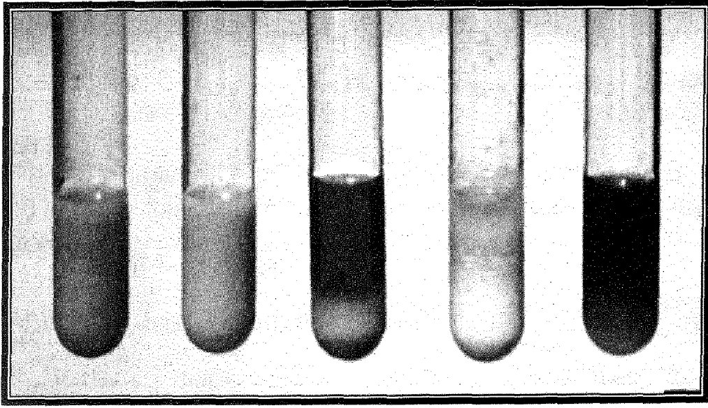
شكل (33) تفاعلات حليب اللتموس.
