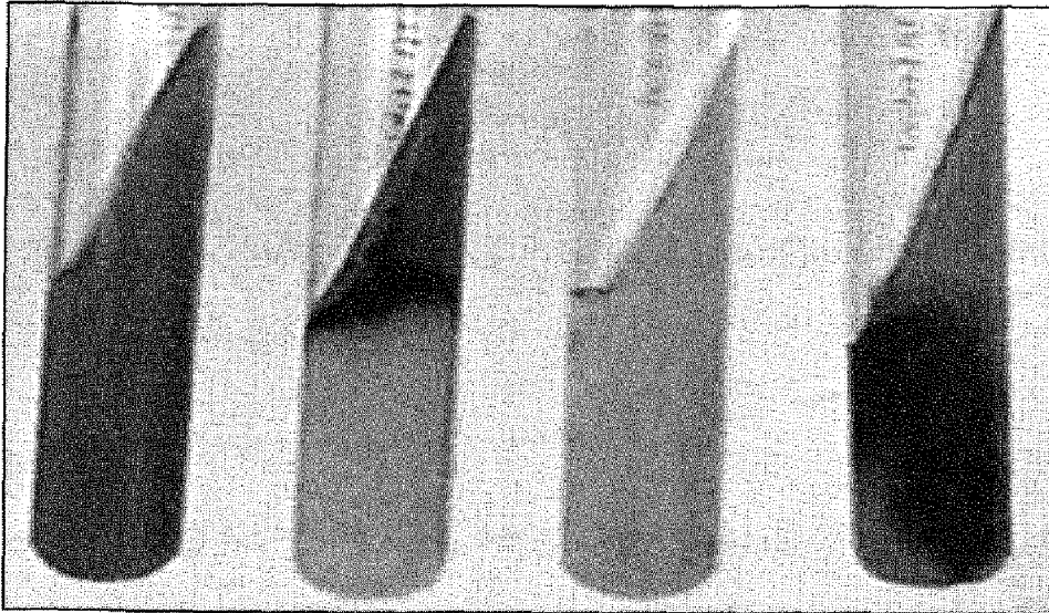
شكل (38) قدرة البكتيريا على تكوين راسب اسود على طول خط الطعن وتكون غاز H_2S
