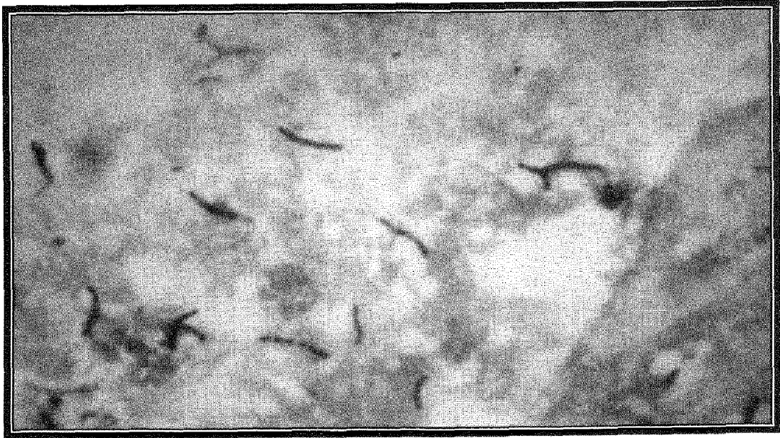
شكل (16) بكتريا Mycobacterium مصبوغه بصبغة Acid-Fast Staining.
