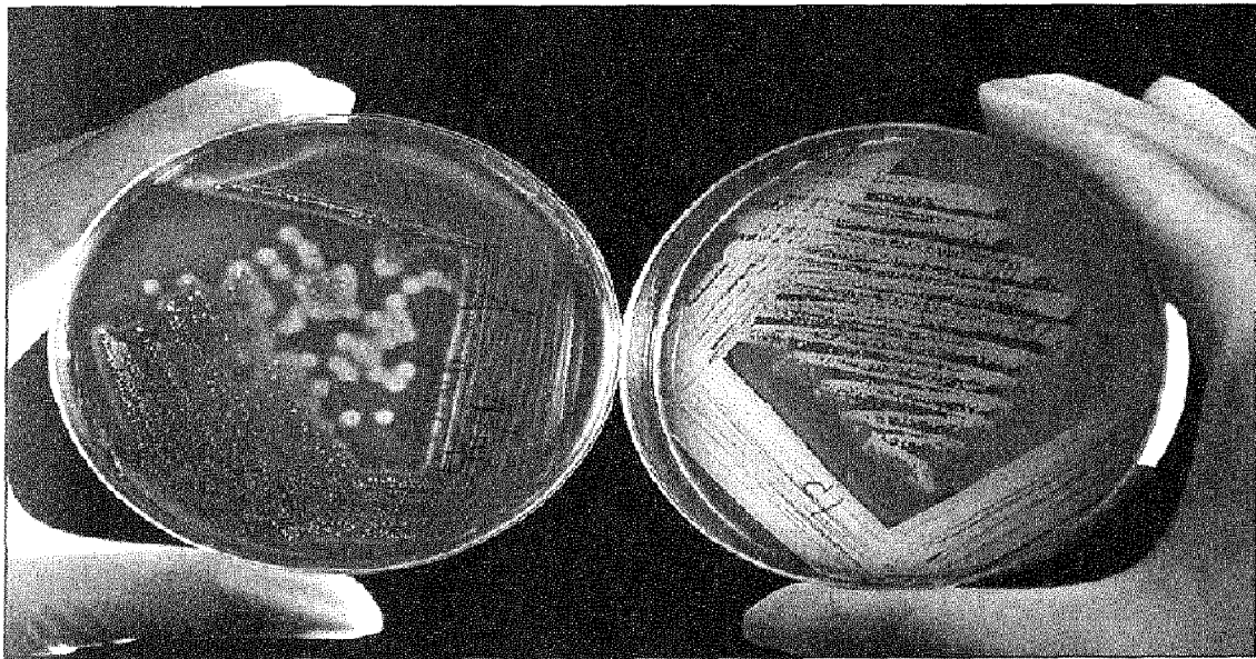
الشكل (12) مزروعة بكتيرية مزروعة بطريقة التخطيط على طبقين زرعين.
