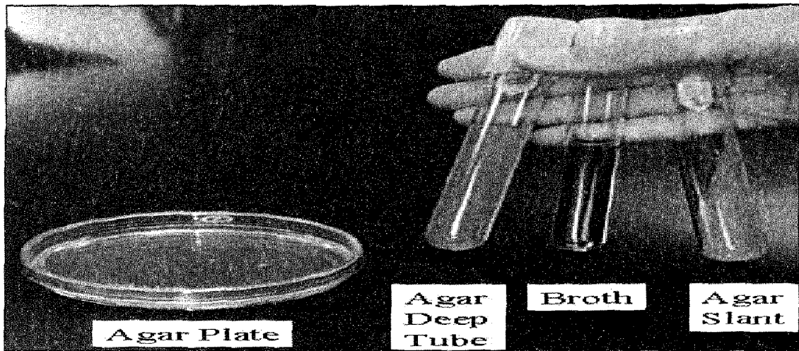
شكل (4) فقسفم الاواسط الزرعفة حسب القوام الى وسط صلب (طبق الاكار) ووسط الاكار السائل.
