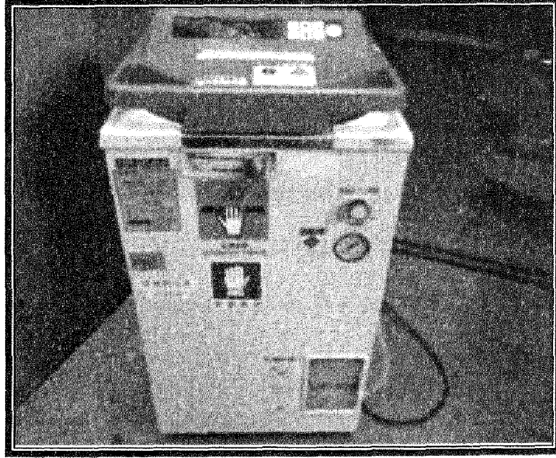
شكل (9) المزارع الميكروبية المراد التخلص منها كمزارع البكتيريا المرضية يتم تعقيمها في الautoclave لمدة 15_20 دقيقة بدرجة حرارة 120 م .
