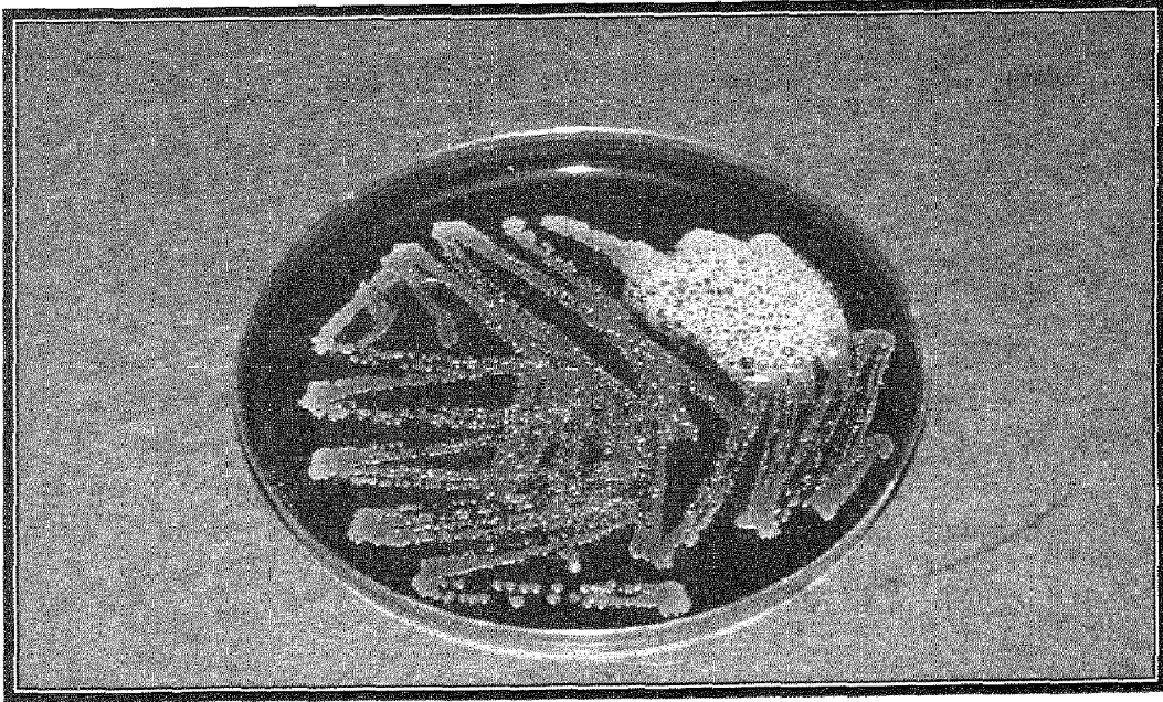
شكل (40) البكتيريا المكورات العنقودية المنتجة للكاتاليز.
