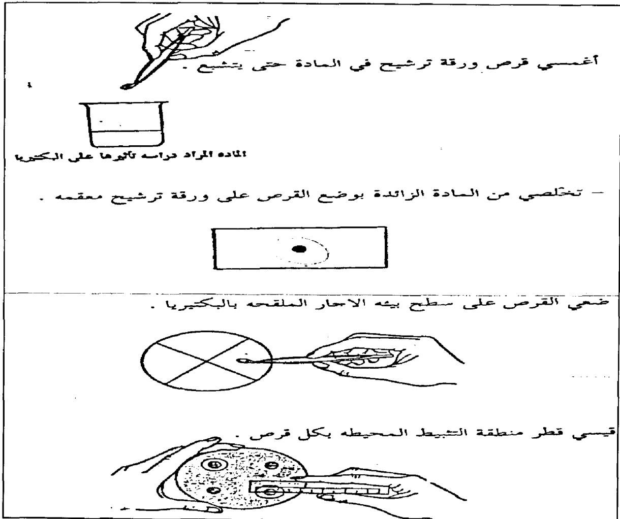
شكل (20) تأثير المضادات الحيويه على البكتريا .
