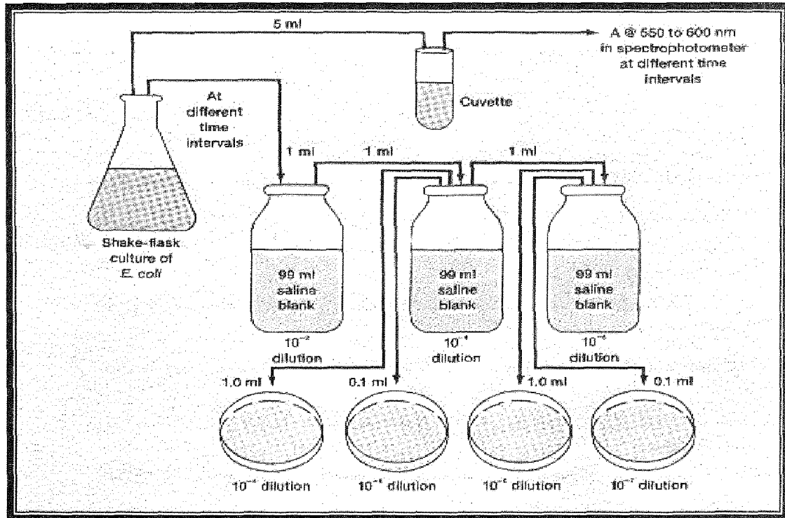
شكل (53) تحديد منحنى النمو في البكتريا مختبرياً
