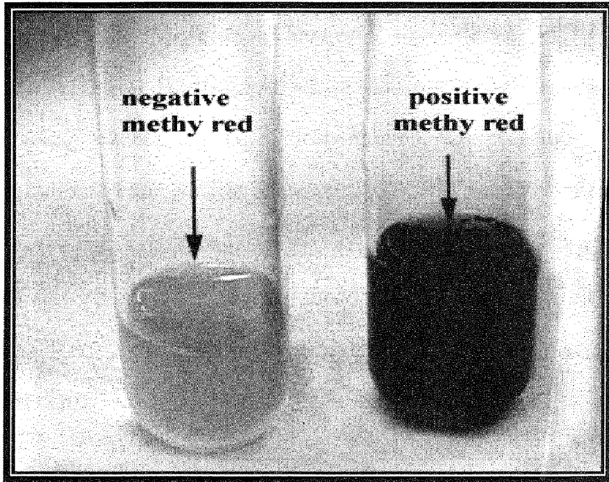
شكل (29) اختبار قابلية بعض البكتريا لتخمير السكريات 1- الفحص الموجب 2- فحص
