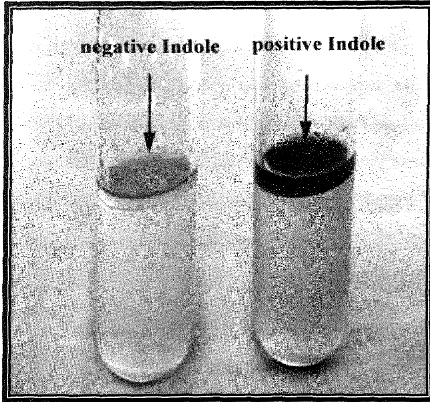
شكل (28) اختبار الاندول 1- الفحص الموجب 2- فحص السالب.
