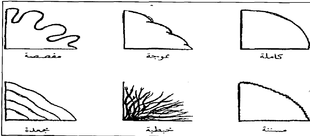
شكل (22) اشكال حافة المستعمرة.
