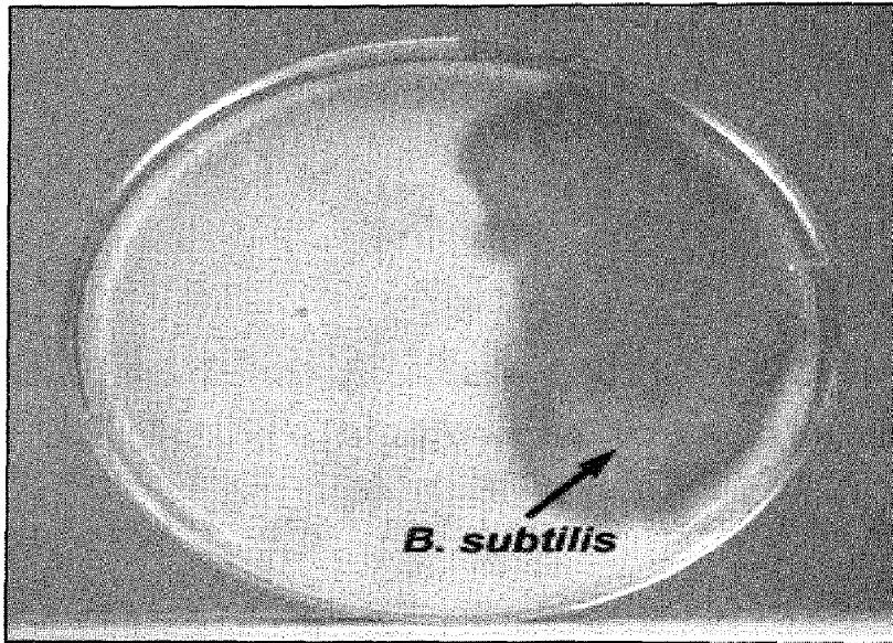
شكل (36) نمو البكتيريا B.subtilis على وسط اكار اللين وتحللها الكازين.
