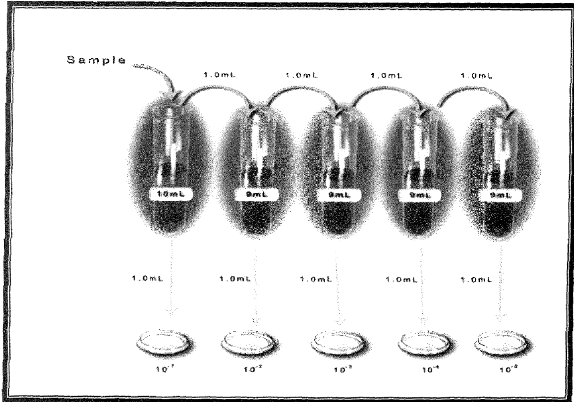
الشكل (27) تقدير عدد الخلايا الحية بطريقة العد بالأطباق Plate Count method
