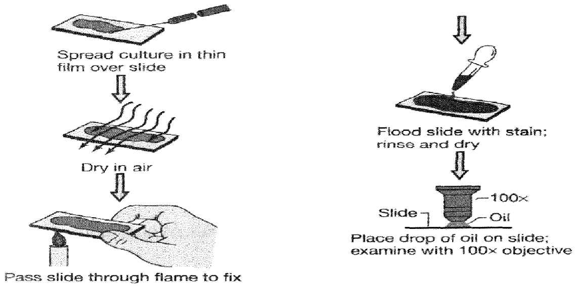
شكل (14) طريقة التصبغ بصيغة كرام .
