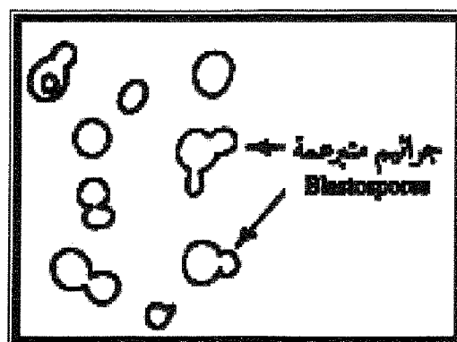
شكل (50) انواع مختلفة من الخمائر تحت المجهر.
