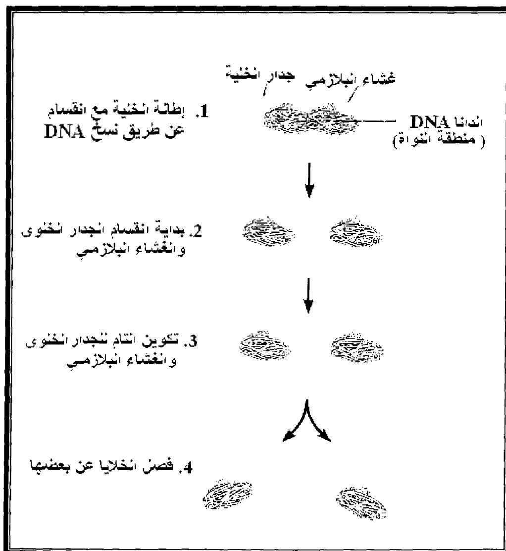
شكل ( 47 ) الانقسام الثنائي البسيط لخلية بكتيرية .
