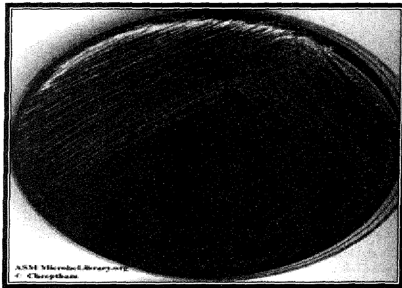
شکل (7) نمو مستعمرات E. coli علی وسط EMB.
