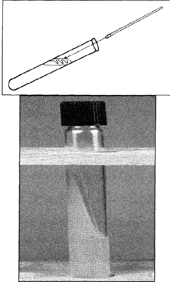
شكل(13) تلقيح سطح الاكار المائل بالبكتيريا.
